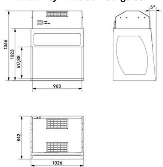
CleanBoy® Plus 56 Tischgerät
