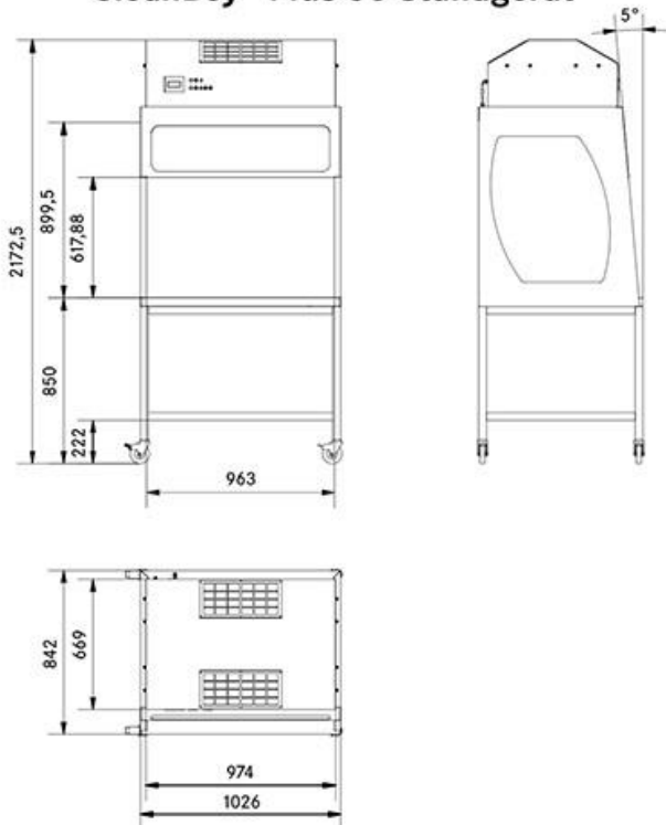
CleanBoy® Plus 56 Standgerät
